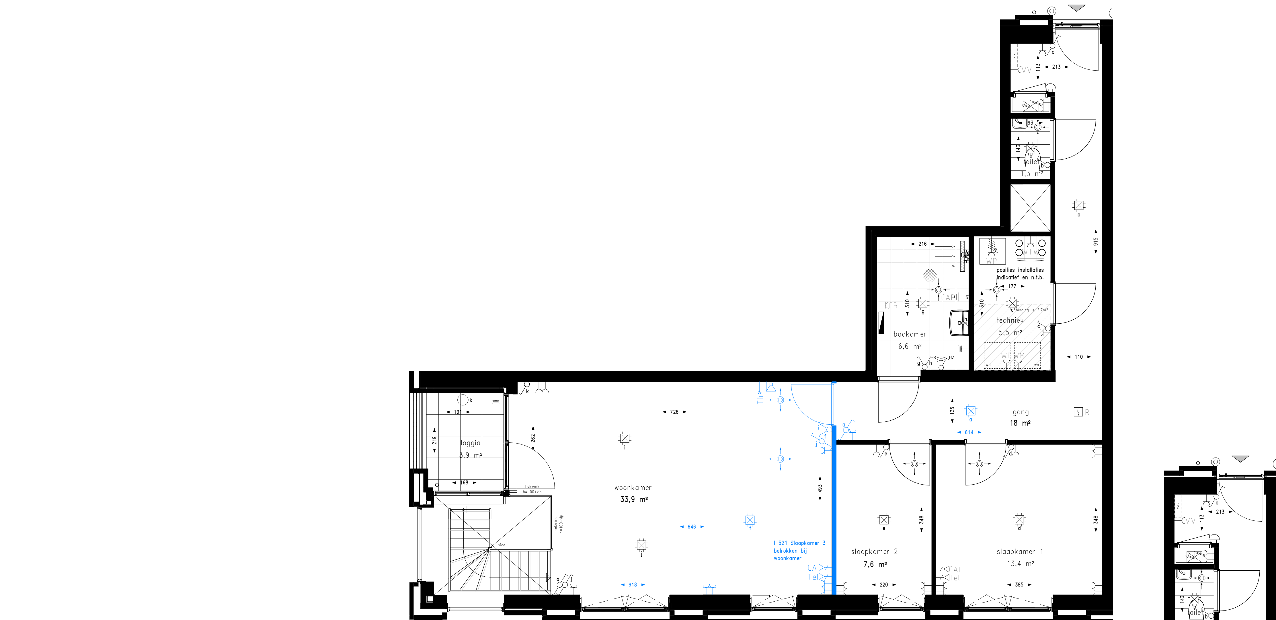
Eerste verdieping
