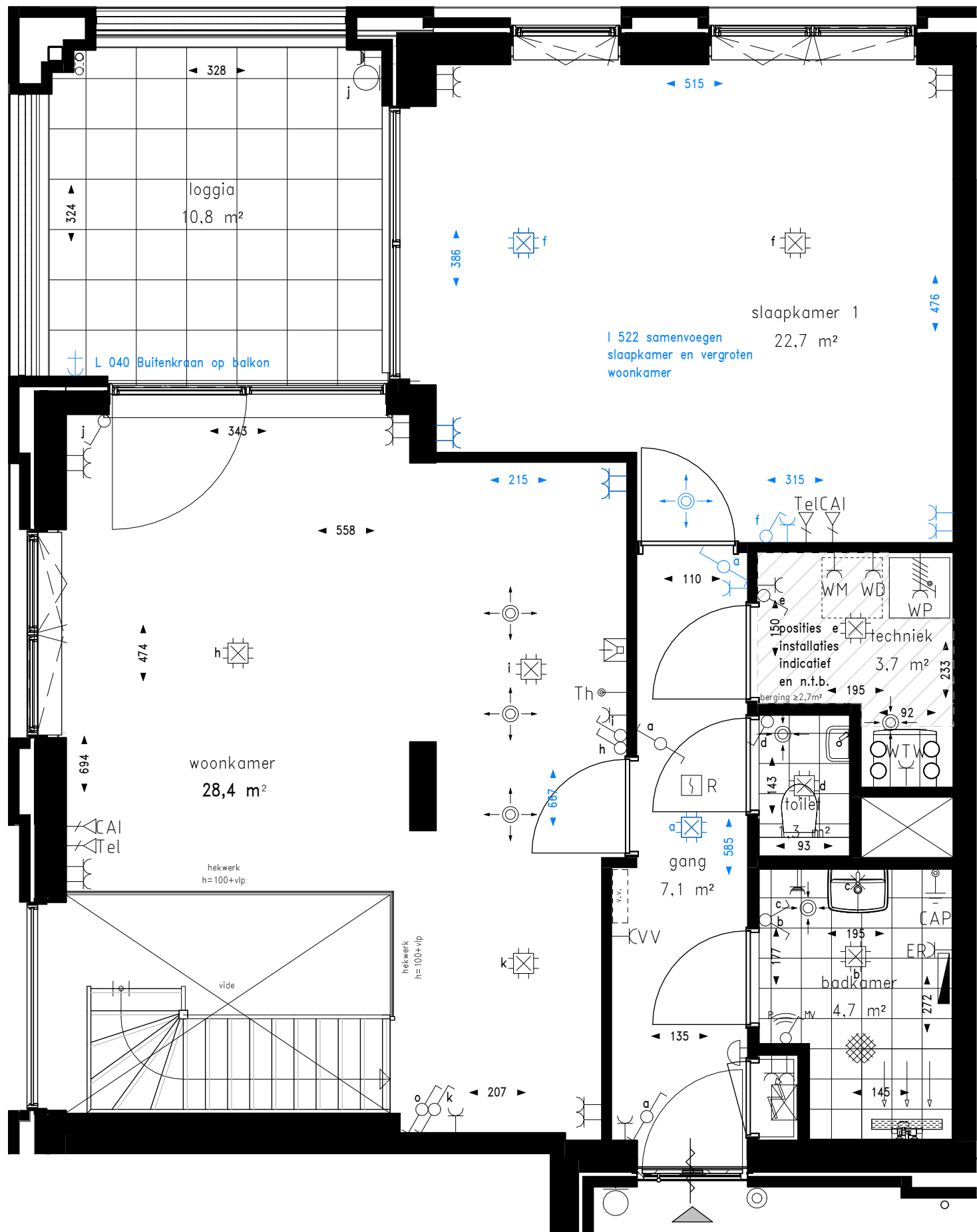
Eerste verdieping
