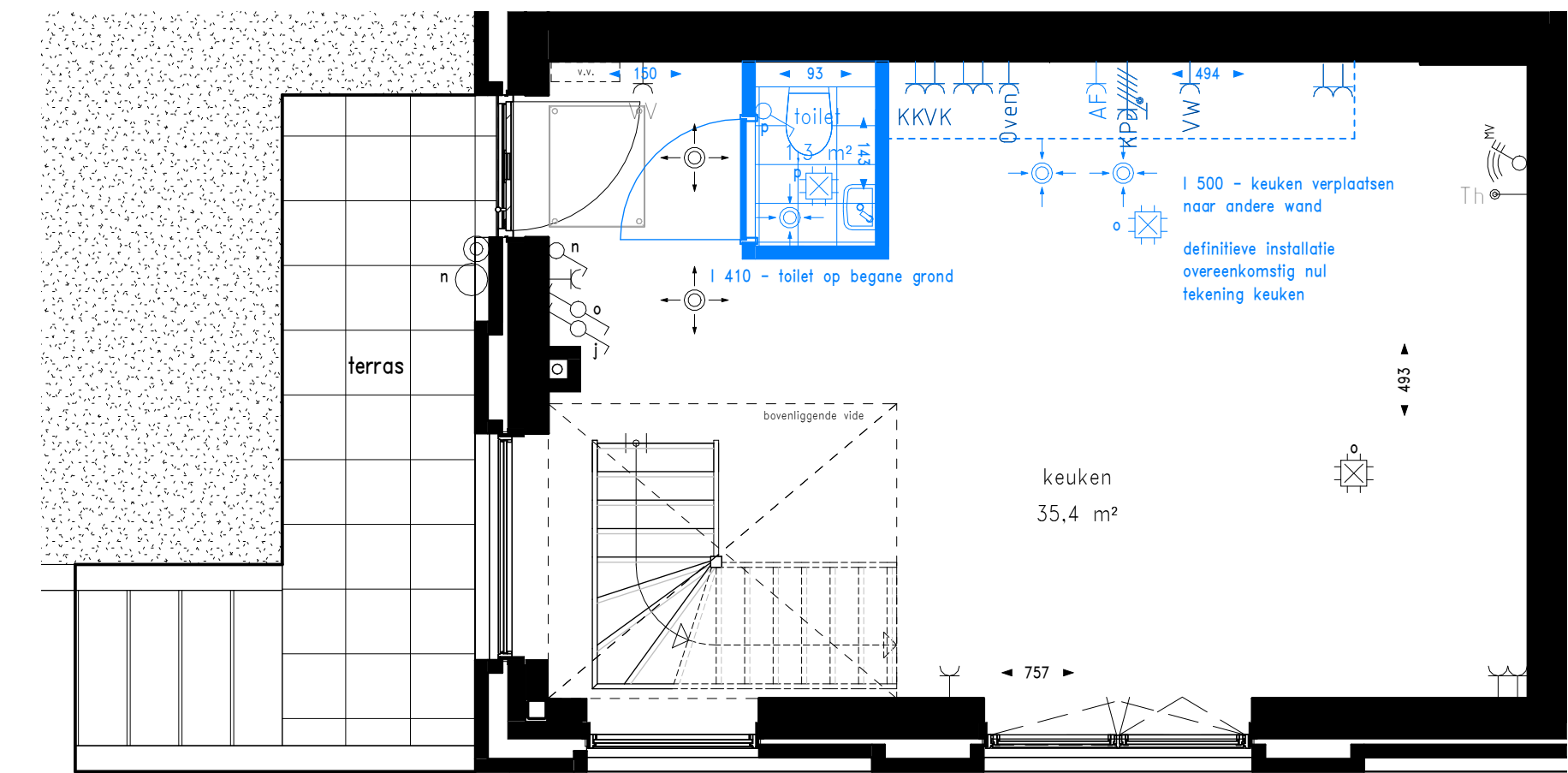
Begane grond
