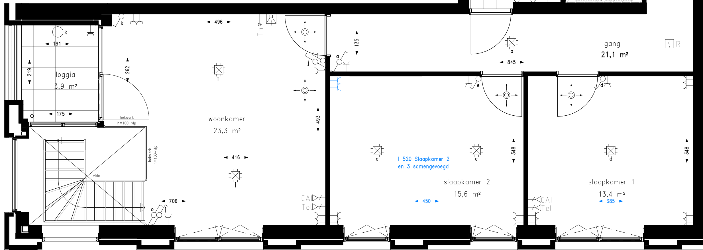
Eerste verdieping
