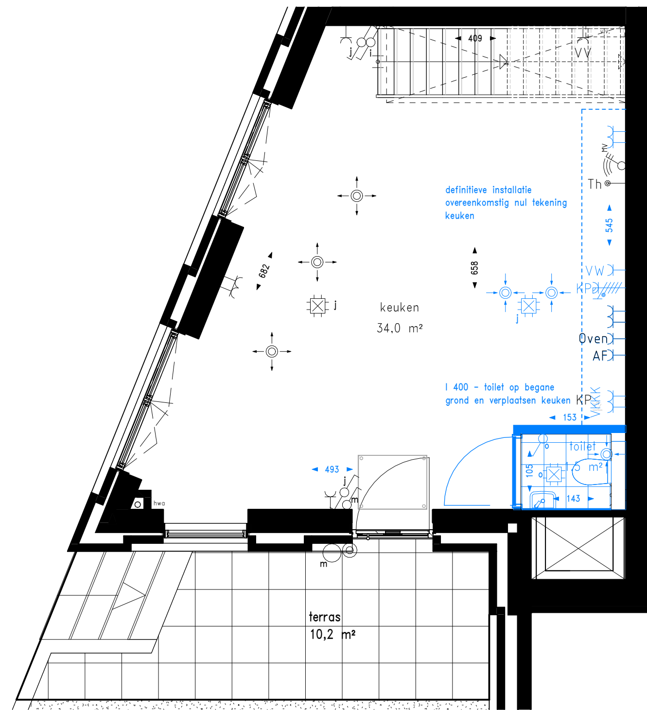
Begane grond
