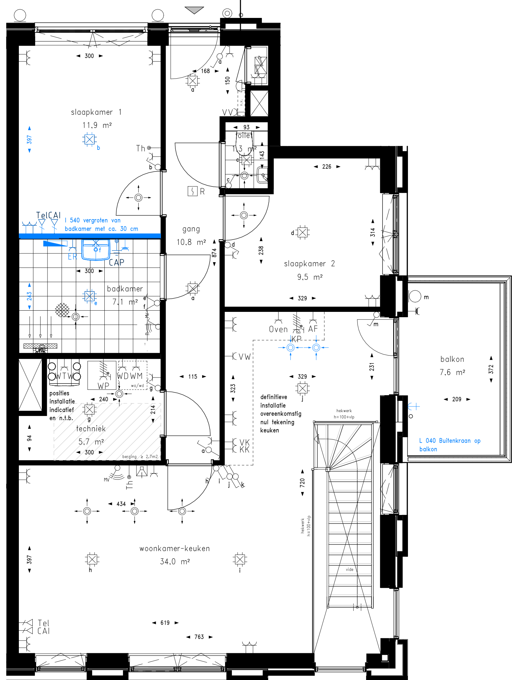
Eerste verdieping
