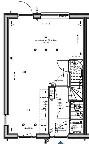
Begane grond
