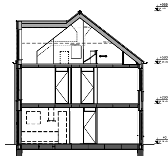
Doorsnede (1:100)
