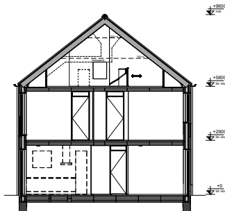
Doorsnede (1:100)
