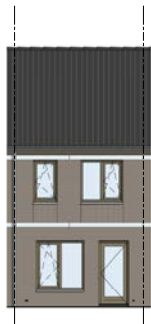
Achtergevel (1:100)
