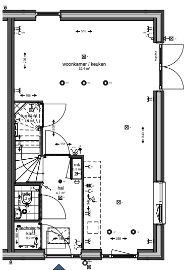
Begane grond
