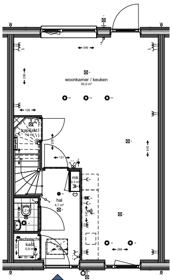
Begane grond
