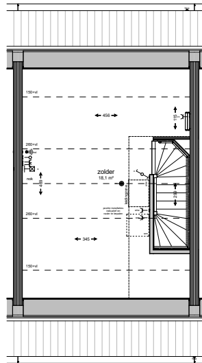
2e verdieping
