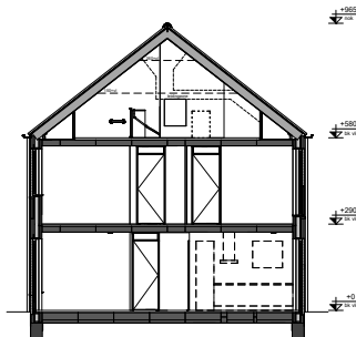
Doorsnede (1:100)
