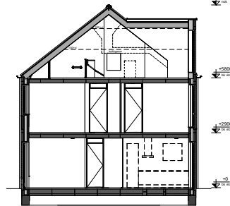
Doorsnede (1:100)
