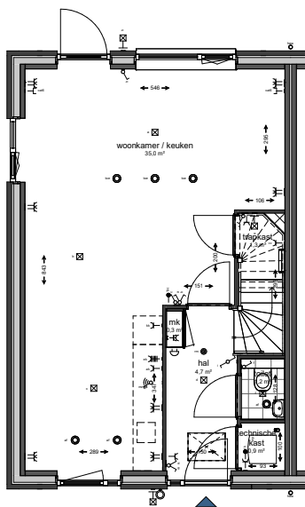
Begane grond
