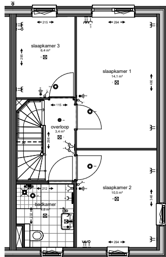
1 e verdieping
