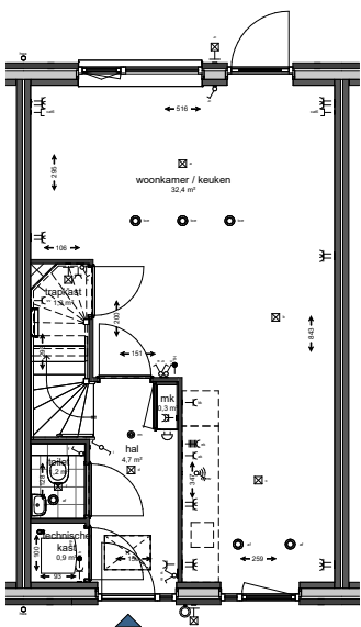
Begane grond
