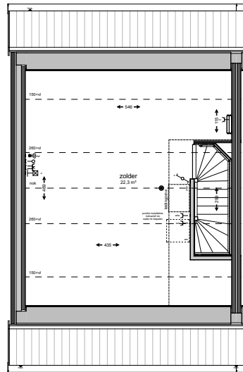
2e verdieping
