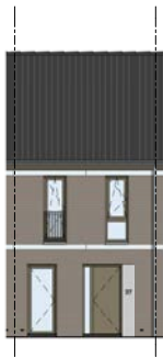
Voorgevel (1:100)
