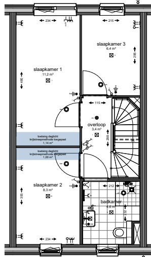
1e verdieping
