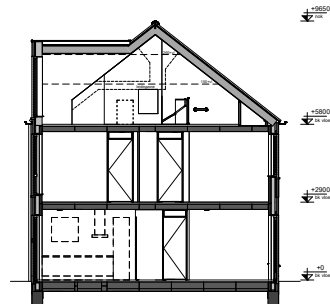
Doorsnede (1:100)
