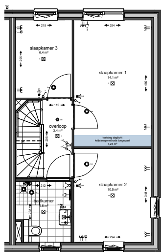
1 e verdieping
