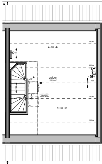
2 e verdieping
