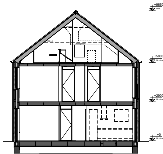
Doorsnede (1:100)
