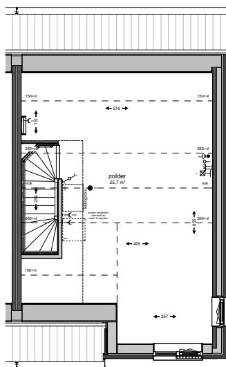
2 e verdieping
