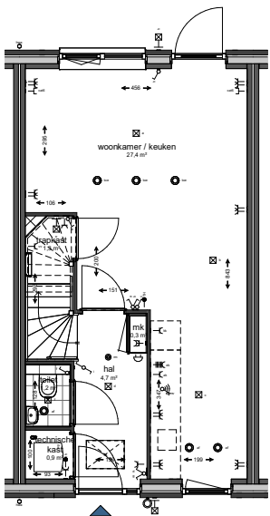
Begane grond
