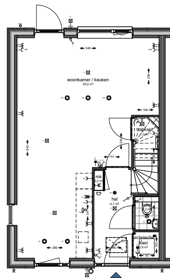
Begane grond
