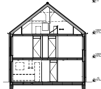
Doorsnede (1:100)
