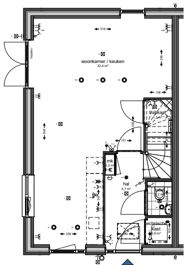
Begane grond
