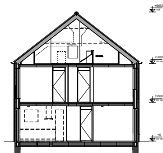
Doorsnede (1:100)
