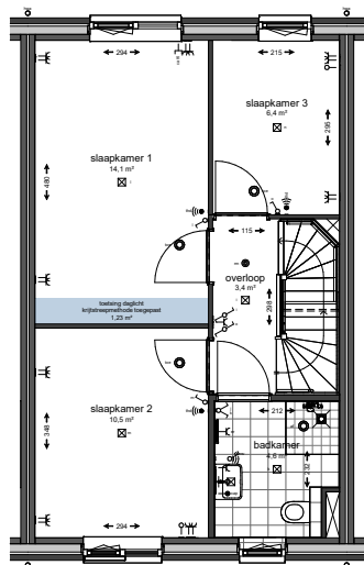
1e verdieping
