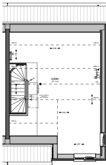
2e verdieping
