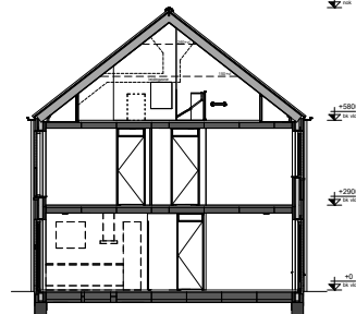
Doorsnede (1:100)
