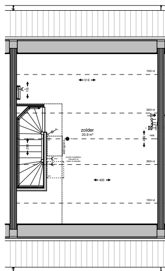
2e verdieping
