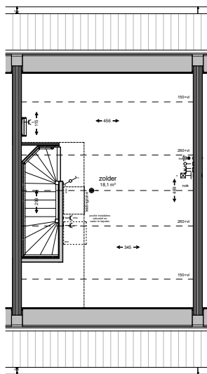
2e verdieping
