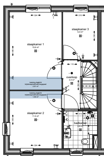
1° verdieping
