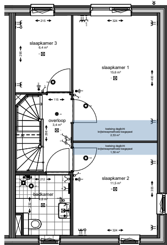
1e verdieping
