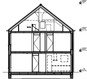
Doorsnede (1:100)
