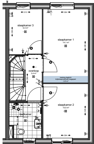
1 o verdieping
