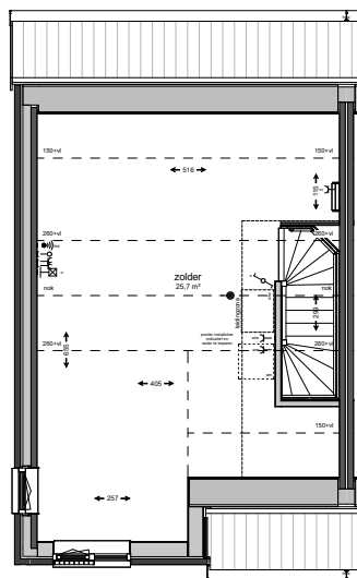
2° verdieping
