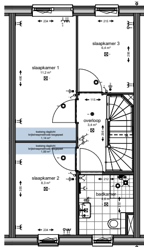
1e verdieping
