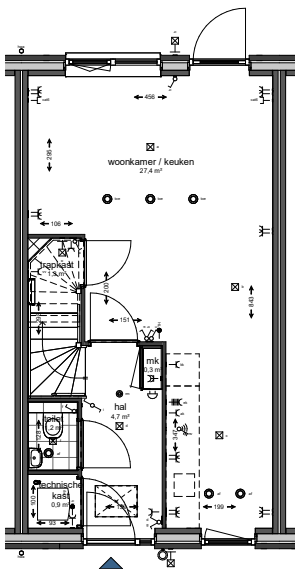
Begane grond
