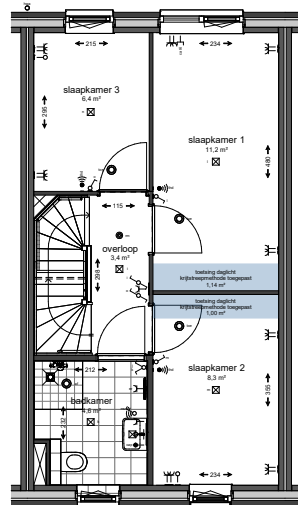
1 e verdieping
