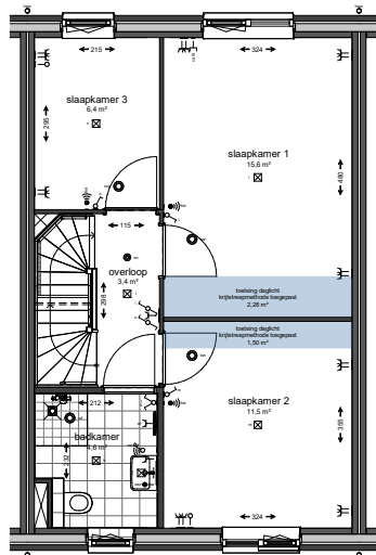
1e verdieping
