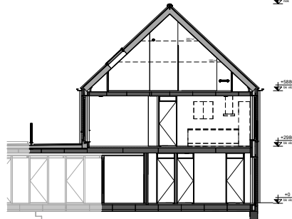
Doorsnede (1:100)
