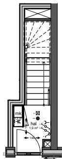
Begane grond
