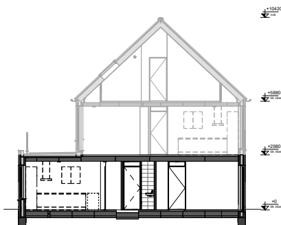
Doorsnede (1:100)
