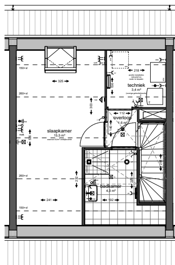
2 e verdieping
