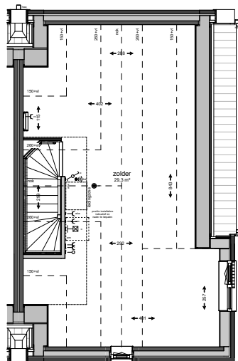
2e verdieping
