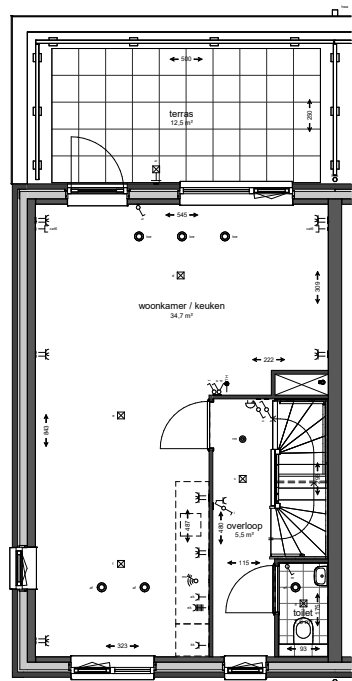
1° verdieping
