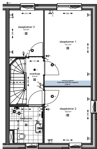
1e verdieping
