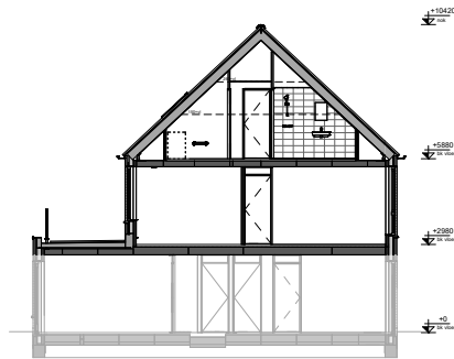
Doorsnede (1:100)
