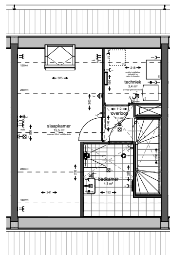
2e verdieping
