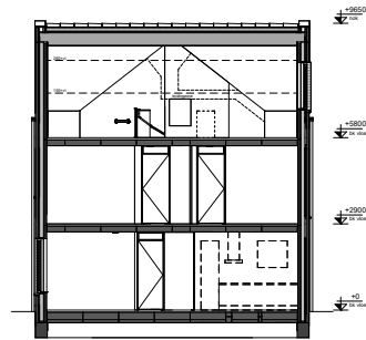
Doorsnede (1:100)
