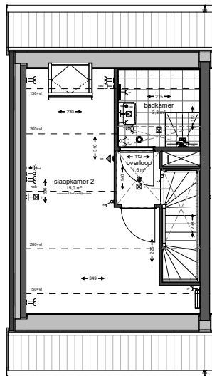
2e verdieping
