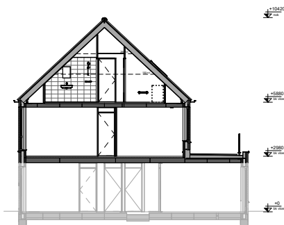
Doorsnede (1:100)
