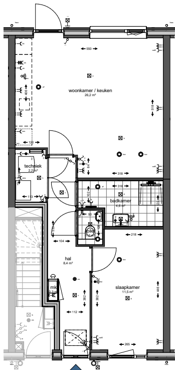
Begane grond
