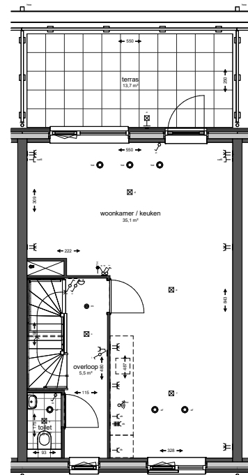
1e verdieping
