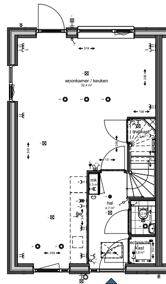
Begane grond
