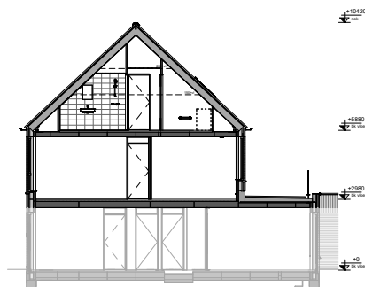
Doorsnede (1:100)
