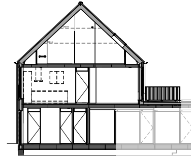
Doorsnede (1:100)
