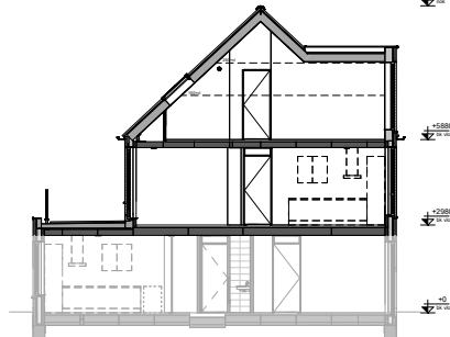
Doorsnede (1:100)
