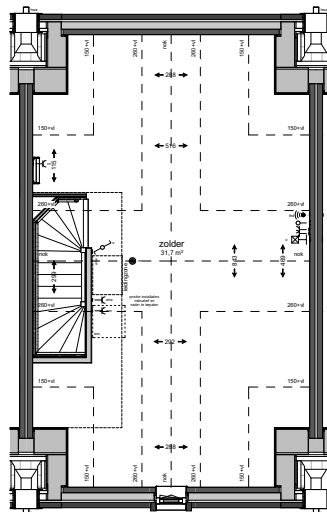
2 de verdieping
