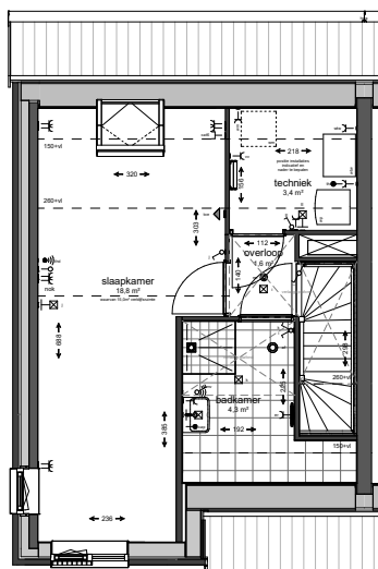
2° verdieping
