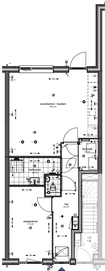
Begane grond
