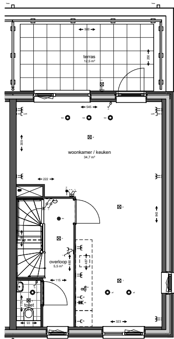
1e verdieping
