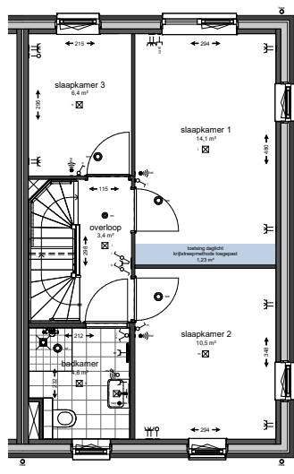
1 e verdieping
