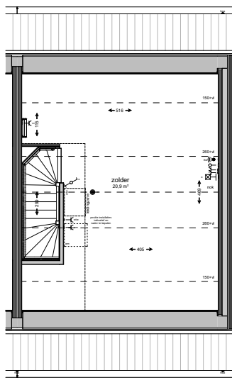
2 e verdieping
