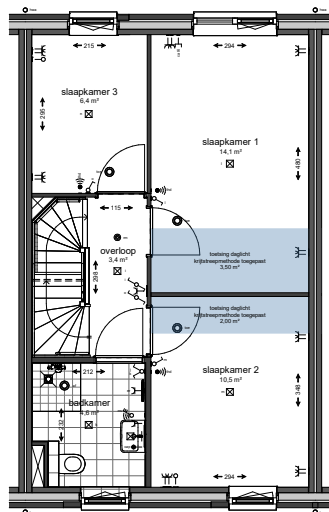
1 ste verdieping
