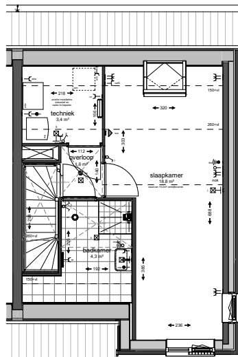
2e verdieping
