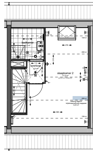
2e verdieping
