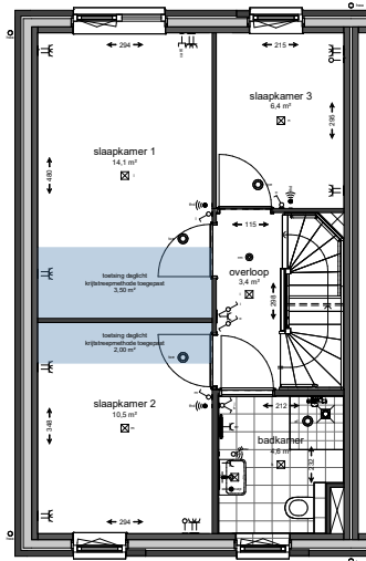
1e verdieping
