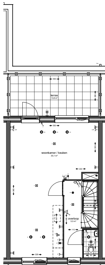
1e verdieping
