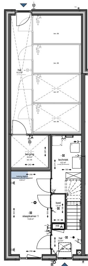
Begane grond
