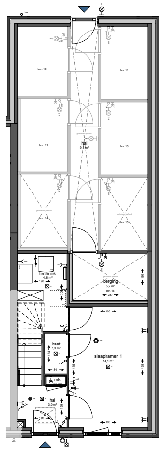
Begane grond
